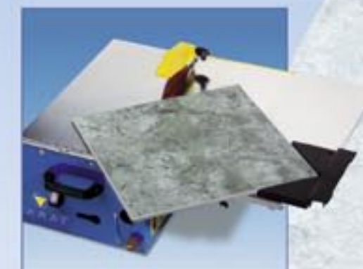
Guide coulissant avec guide diagonal
