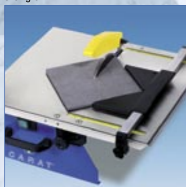
Guide réglage pour les coupes en diagonal
